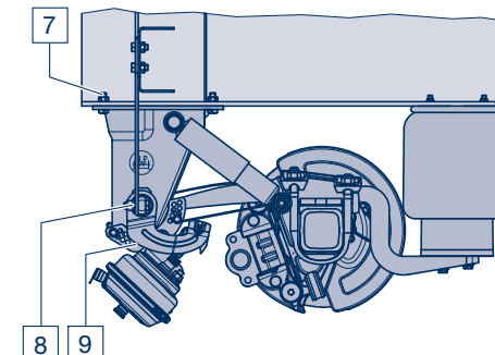
Серия ALM/SLM с привинчиваемым кронштейном
