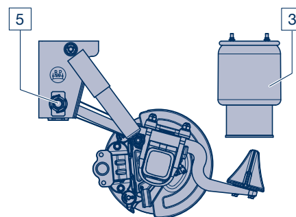
Серия ALM/SLM с комбинированной рессорой Kombi-Air Bag II
